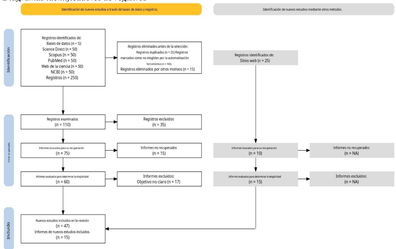
Figura 1 Diagramas identificadores de registros
