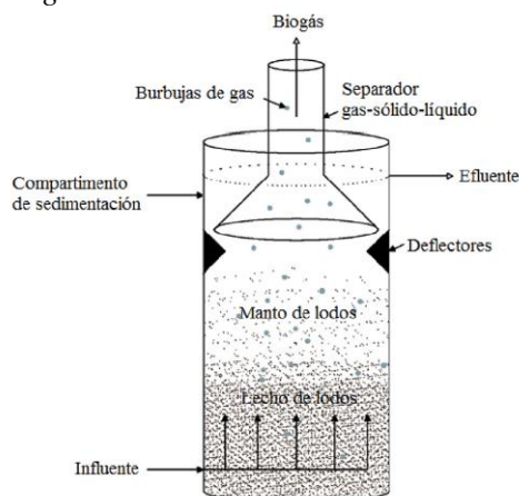
Diagrama de Reactor UASB
